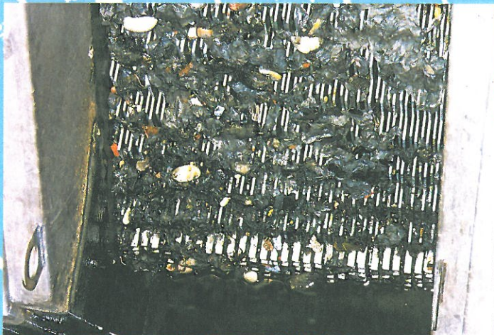
Optimaalinen askellus nostaa ja siirtää erottuvan välpeen tehokkaasti välpepuristimeen
